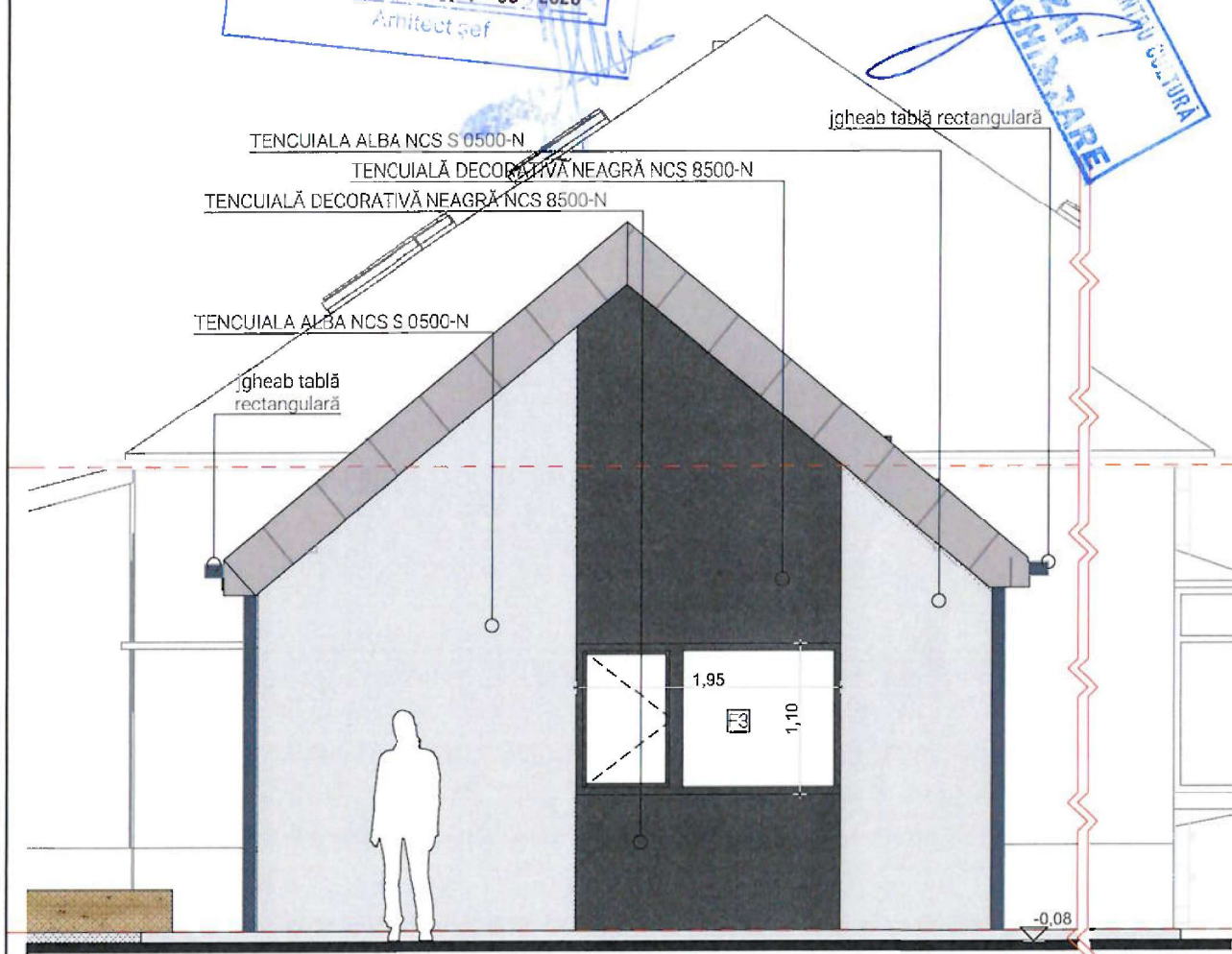
FN Fatada Nord SCARA 1:50
